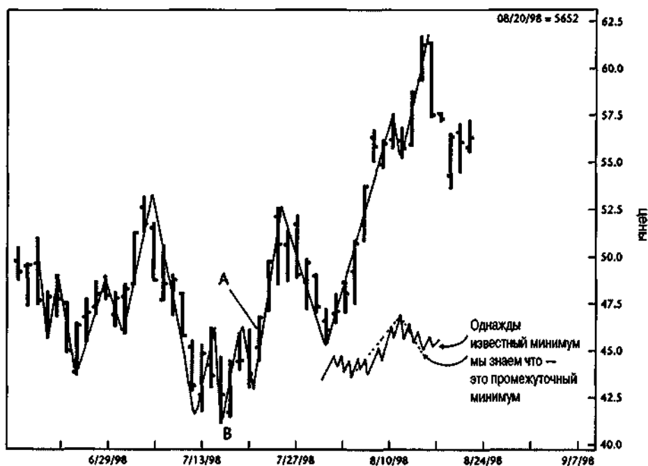
Рисунок 1.10 Свирина (дневные бары). График создан программой «Navigator» (Genesis Financial Data Services).
